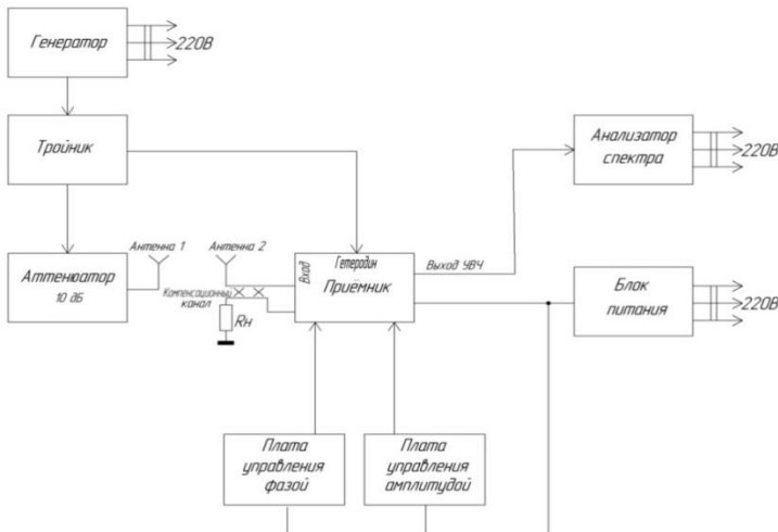
Рисунок 7. – Структурная схема измерений величины подавления сигнала при коммутации через эфир
